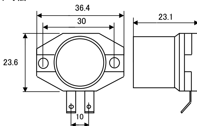
図1 形状・寸法
